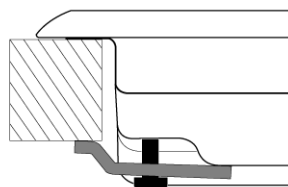
Положение фиксатора при H = 30 \text{ мм}
