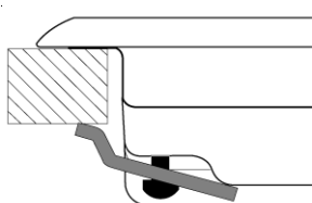
Положение фиксатора при H^* = 20 \text{ мм}
